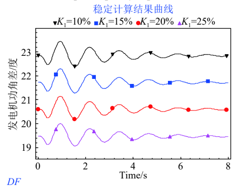
图 11 DF 风机等容量替换发电机功角差
