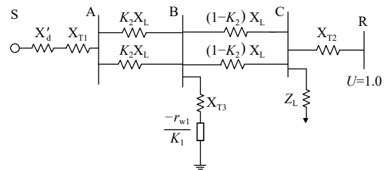
图 2 稳态运行时系统的等值电路
